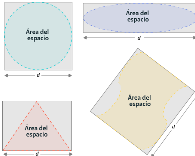
Figura 4.3.9.1. a. Ejemplos de determinación del área de la malla de medición (Fuente propia).
