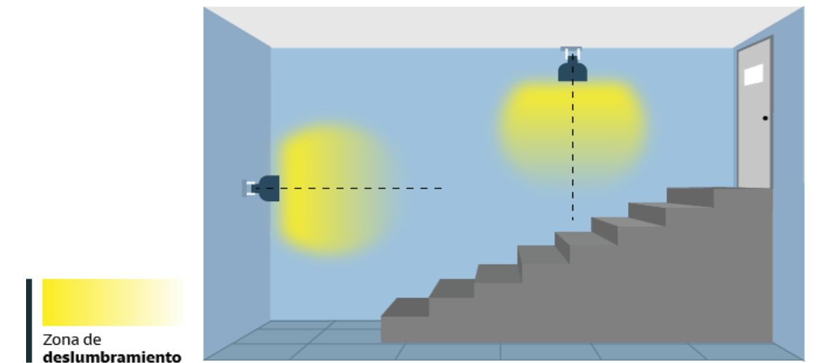
Figura 3.2.4. c. Zonas de deslumbramiento en zonas de énfasis, antipánico, áreas de alto riesgo. (Adaptado de NTC 6556)
