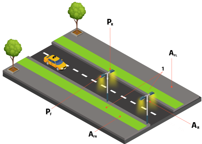
Figura 3.3.1.8. a. Ejemplo perfil vía para calculo PDI(Dp) y AECI(DE). (Fuente propia)
