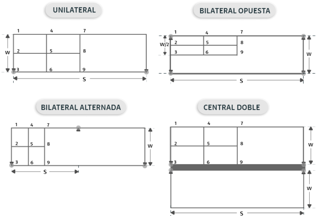
Figura 4.3.11.1 b. Selección de los 9 puntos según disposición de las luminarias (Adaptada del RETILAP 2010).
