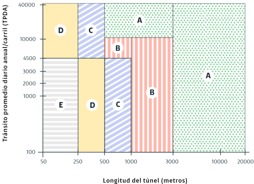
Figura 3.5.4. a. Clasificación de túneles viales por longitud y TPD en Colombia (Adaptada de: Manual para el diseño, construcción, operación y mantenimiento de túneles de carretera para Colombia –INVIAS 2021).
