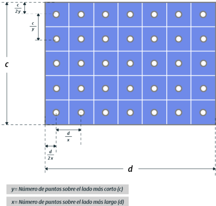
Figura 4.3.9.1. c. Relaciones de la distancia entre puntos de una malla típica (Adaptada de BS EN 12464-1).
