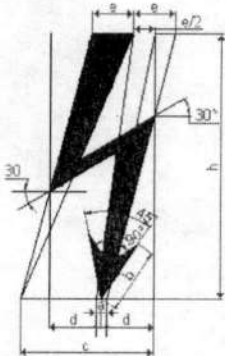
Figura 4. Símbolo de riesgo eléctrico
