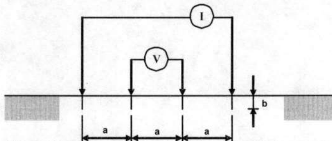
Figura 13. Esquema de medición de resistividad aparente.
