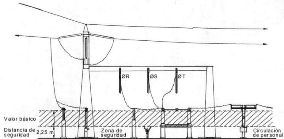
Figura 20. Zona de seguridad para circulación de personal
