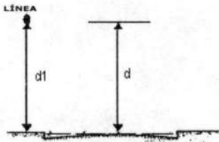
Figura 6. Distancias “d” y “d1” en cruce y recorridos de vías
