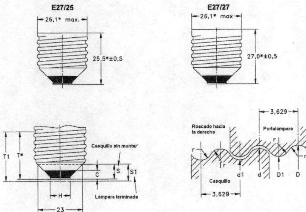
Figura 17. Dimensiones del casquillo de una bombilla en milímetros.
