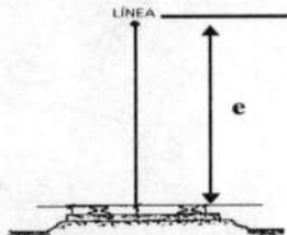
Figura 7. Distancia “e” en cruces con ferrocarriles sin electrificar
