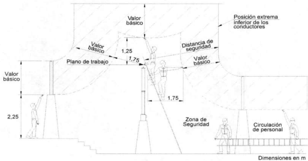
Figura 21. Zonas de seguridad
