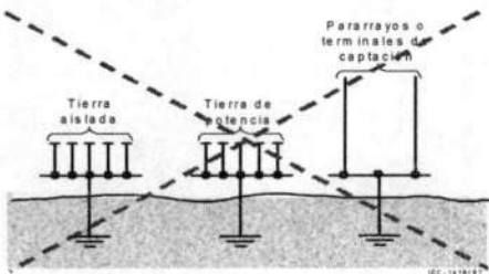
Figura 12. Puestas a tierra separadas e independientes
