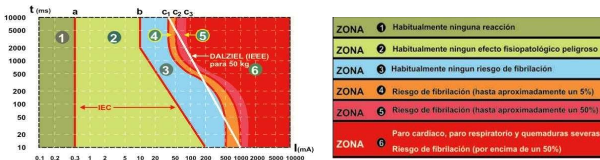
Figura 1.6.1 Zonas de tiempo/corriente de los efectos de las corrientes alternas de 15 Hz a 100 Hz
