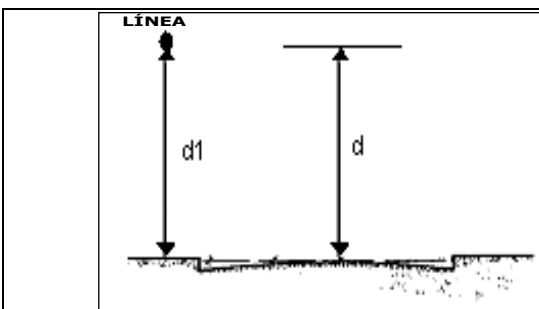
Figura 11.2.1. Distancias “d” y “d1” en cruces y recorridos de vías
