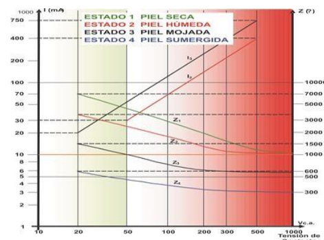
Figura 1.6.2. Impedancia del cuerpo humano
