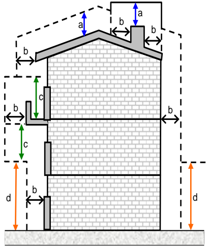
Figura 11.1.1. Distancias de seguridad en zonas con construcciones
