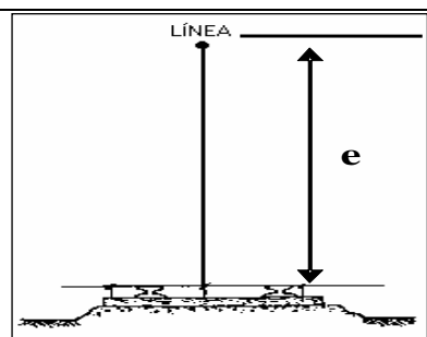
Figura 11.2.2. Distancia “e” en cruces con ferrocarriles sin electrificar
