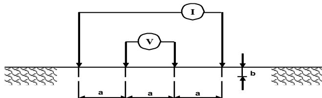
Figura 13.4.1.1. Esquema de medición de resistividad aparente
