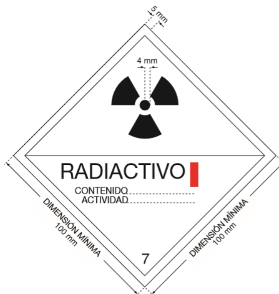
Figura 2: Etiqueta para la categoría I-BLANCA. La anchura mínima de la línea dentro del borde que forma el rombo será de 2 mm. El color de fondo de la etiqueta será blanco, el trébol y los caracteres y líneas impresos serán negros y la barra que indica la categoría
