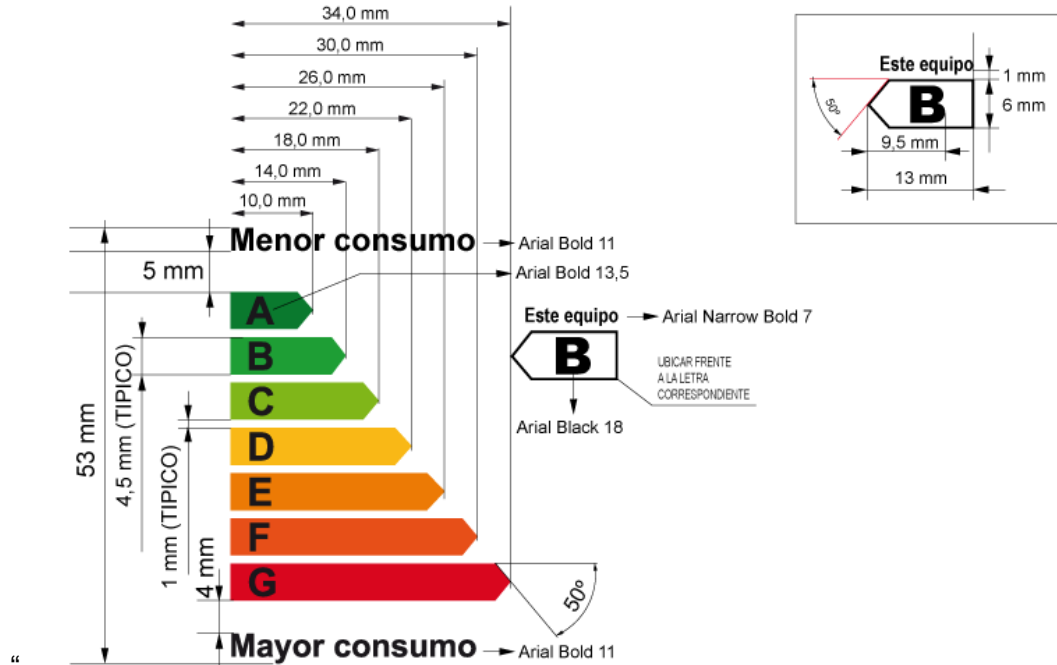
Figura 6.3.3.1. Especificaciones para la ilustración de rangos de eficiencia con barras de colores en tamaño de etiqueta A6 (Dimensiones en milímetros).”
