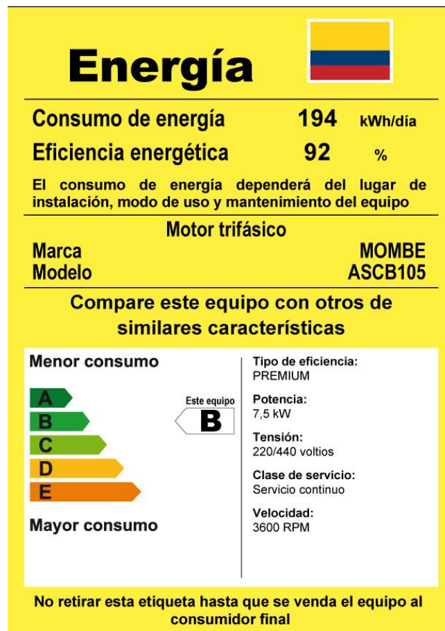
Figura 12.6. Ejemplo de etiqueta para Motores Trifásicos.
